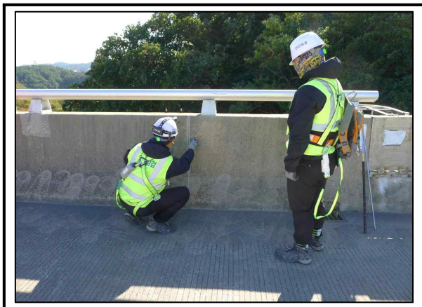
사진번호 55 도보로 상부(방호벽) 외관망도 - 외관조사현황
