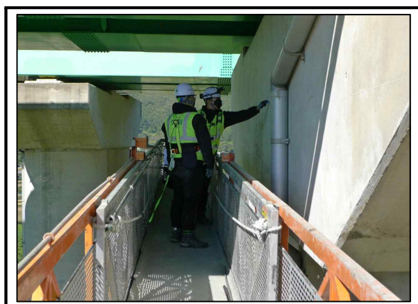
사진번호 60 교량점검차량을 이용한 외관망도 - 외관조사현황
