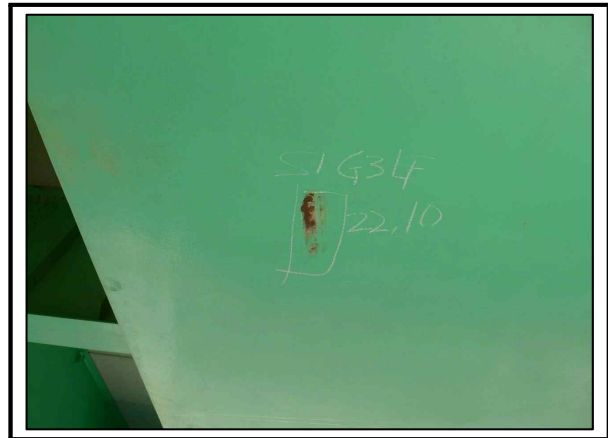
사진번호 26 거더외부 S1 G3 LF 외관망도 80-2 도장긁힘 및 부식
