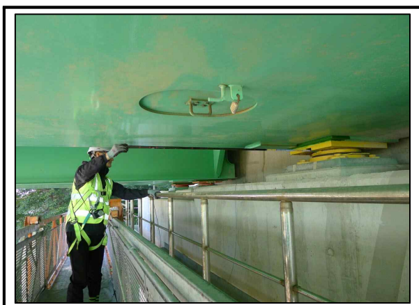
사진번호 57 교량점검시설을 이용한 외관망도 - 외관조사현황
