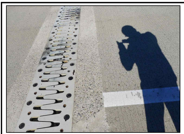
사진번호 21 신축이음 P3 후타재 마모 외관망도 58-3
