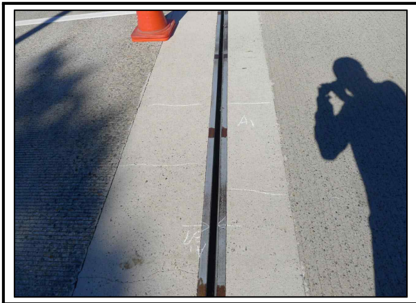
사진번호 19 신축이음 A1 후타재 균열(0.3mm 미만) 외관망도 56-1
