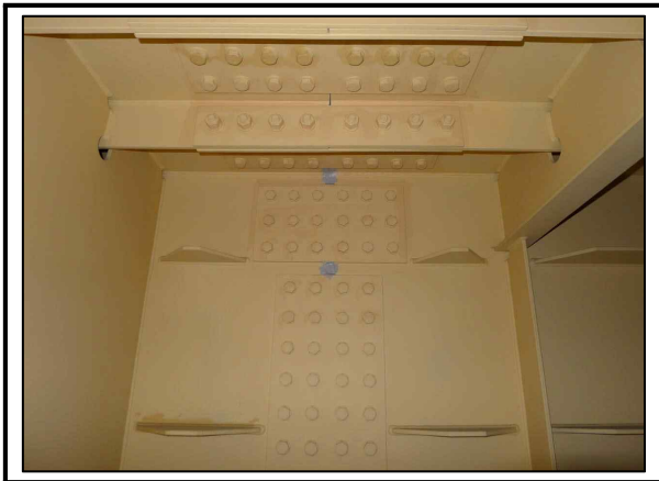
사진번호 31 거더내부 S1 G3 외관망도 - 볼트체결부 실링처리 현황
